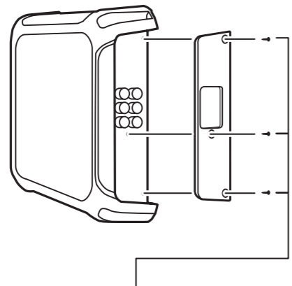
Vis mécaniques (3 mm × 10 mm)
